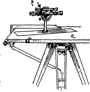
(?) Alidade : दर्शरेखक
